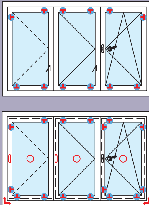
Schematische Zeichnungen
